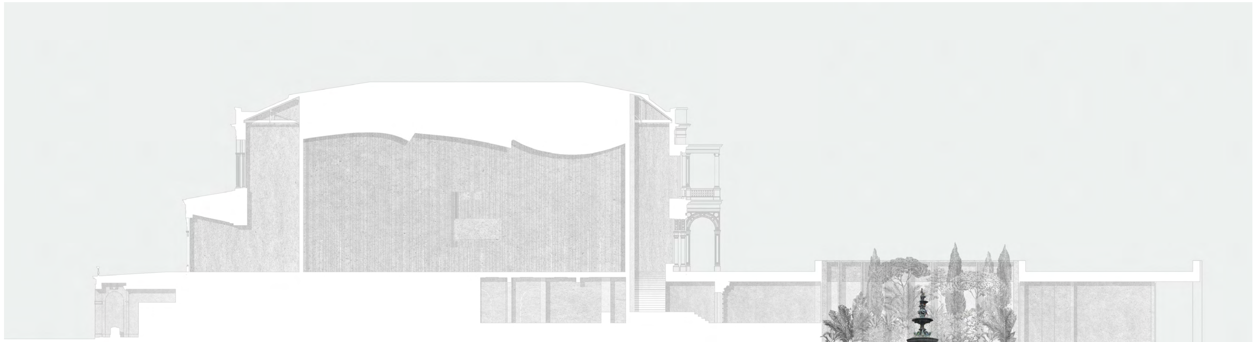
SCHNITT A-A ; M 1:200
