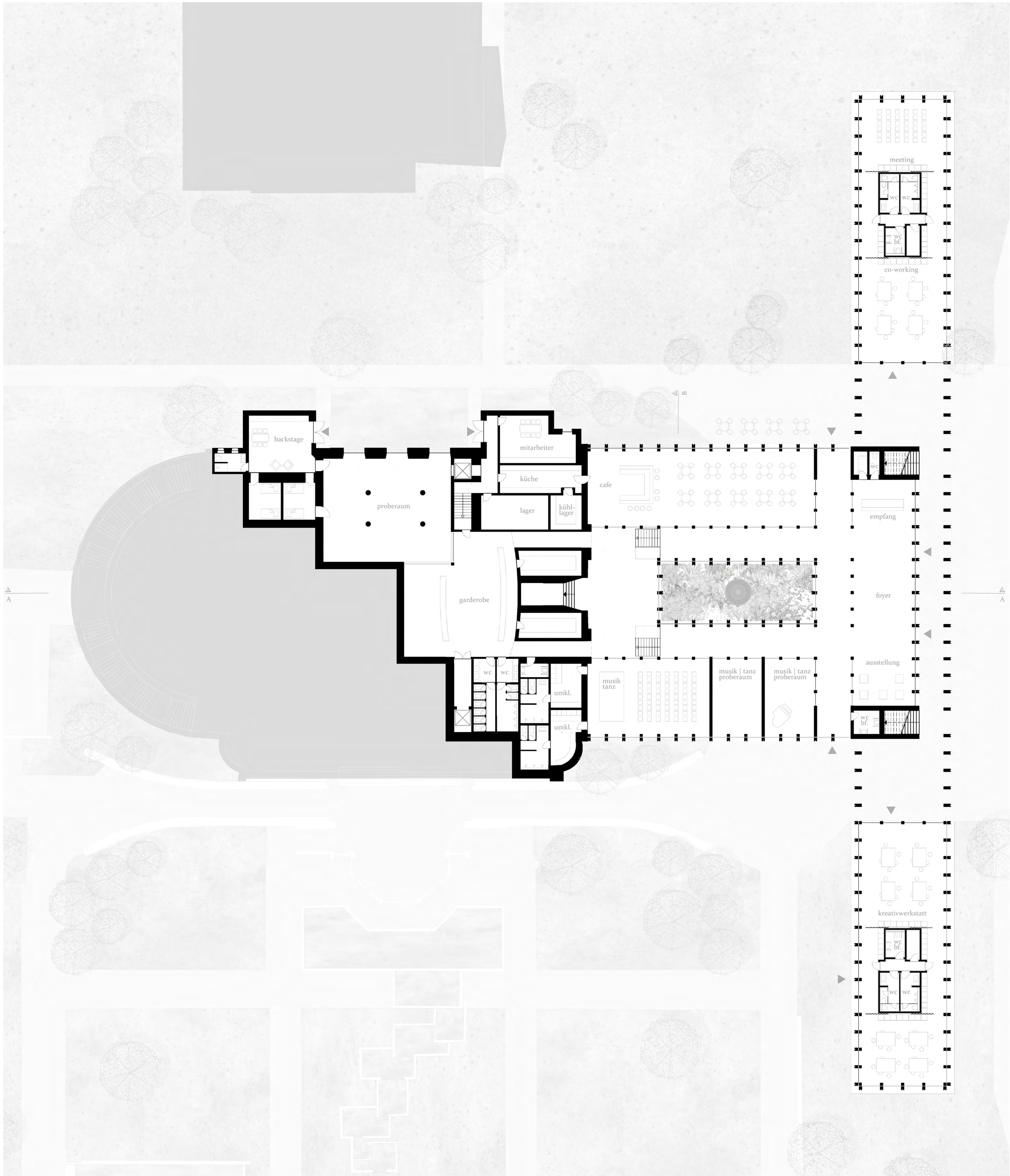
GRUNDRISS E0 | SOCKEL ; M 1:200
