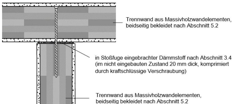
Prinzipskizze 8a: Anschluss Trennwand / Trennwand, Bauteilfuge (Horizontalschnitt)
