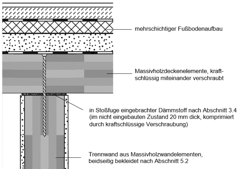
Prinzipskizze 8c: Anschluss Trennwand / Massivholzdecke, Bauteilfuge (Vertikalschnitt)
