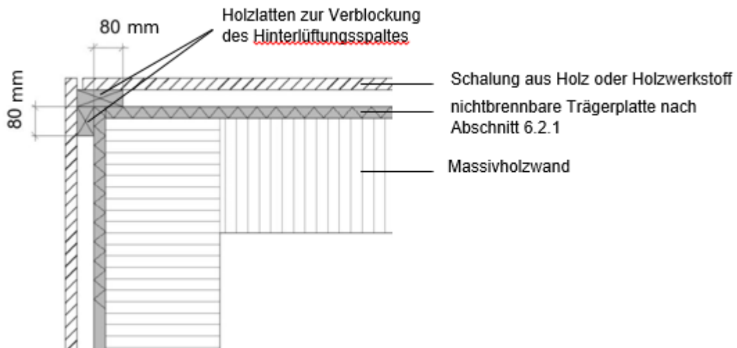
Prinzipskizze 13: Ausbildung Außenwandbekleidung bei Außenecken (Horizontalschnitt)
