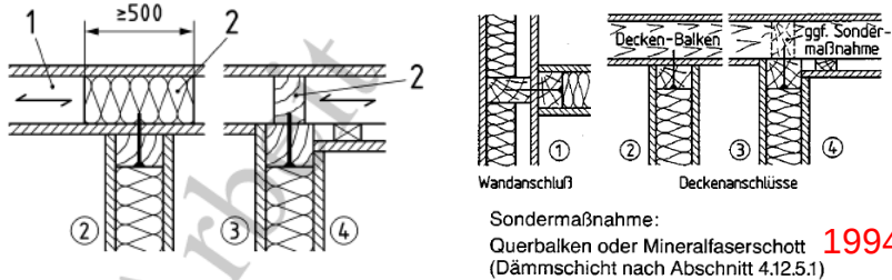
Bild 42: Anschlüsse an Holzbauteilen (Schema)
