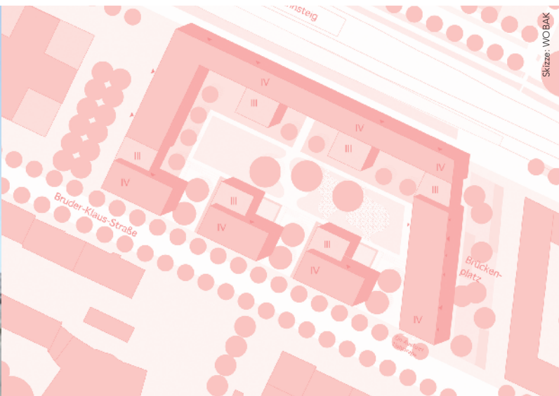
Ein Gebäudeblock schirmt den Bahnlärm ab, die gegenüberliegende Seite ist offen gestaltet.
