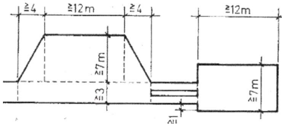
Bild 3: Bewegungsflächen
