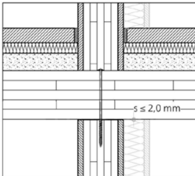
Abbildung 16: Trennwand-Deckenanschlüsse Massivholzbau mit Spaltmaß s \leq 2,0 mm
