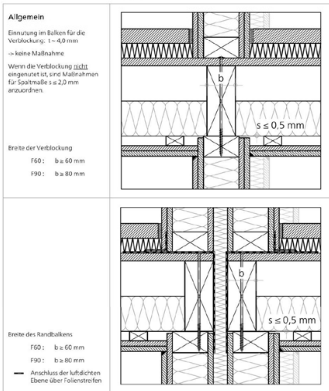
Abbildung 6: Trennwand-Deckenanschlüsse Holztafelbau mit Spaltmaß s \leq 0,5 \text{ mm}
