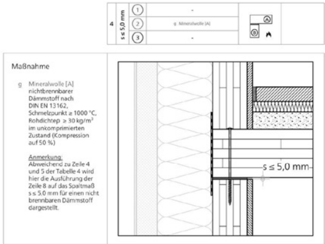
Abbildung 20: Außenwand-Deckenanschluss Massivholzbau mit Spaltmaß s \leq 5,0\text{ mm}
